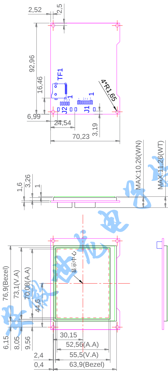
正面视图
